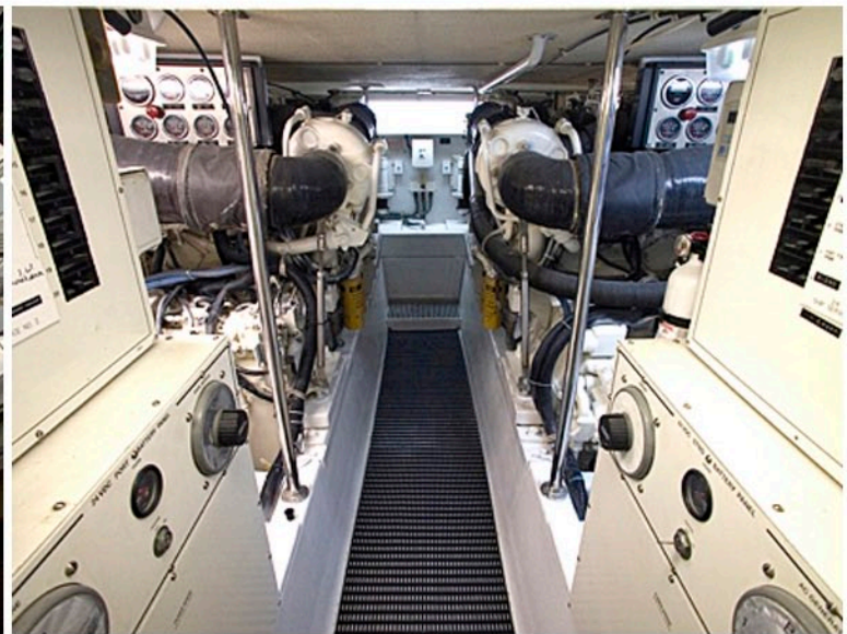
engineroom1.jpg
